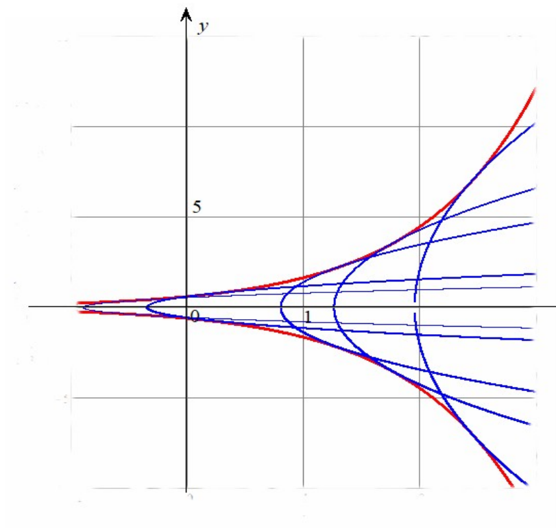
Рис. 1.4. Интегральные кривые для уравнения в задаче 1.5.1
