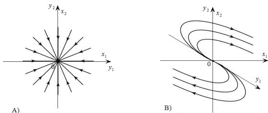
Рис. 6.5. Положения равновесия: дикритический узел и вырожденный узел
