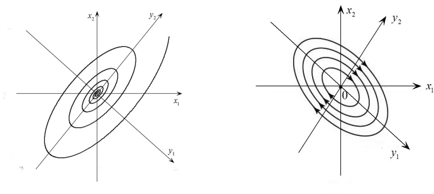
Рис. 6.6. Положения равновесия фокус и центр
