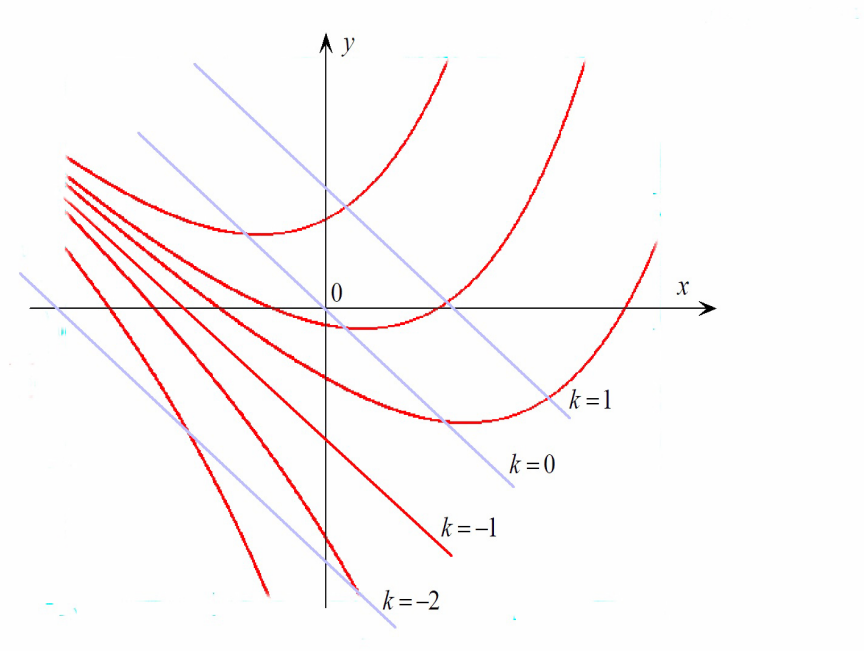
Рис. 1.2. Эскиз семейства интегральных кривых задачи 1.1.1
